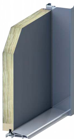
54 AKUSTYCZNE (wewnętrzne)
