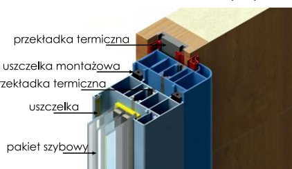
PROFIL NAŚWIETLA PROFIL OŚCIEŻNICY ALU/75
