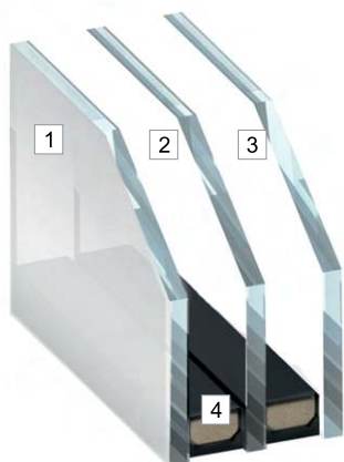
BUDOWA PAKIETU SZYBOWEGO LOFT:
