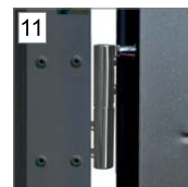
11 Trzy zawiasy 3D z nasadką, regulowane w trzech płaszczyznach
