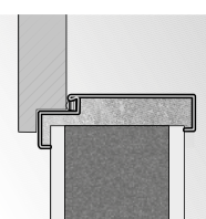
montaż bez dodatkowych elementów kotwiących
