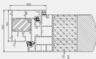
OŚCIEŻNICA
