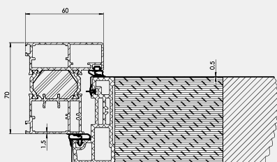
OŚCIEŻNICA
