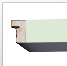
Skrzydło stalowe z wzmocnieniem drewnianym i wypełnione wełną mineralną
